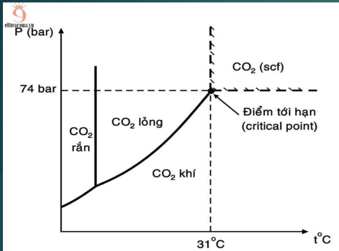
Giải đồ pha CO 2
